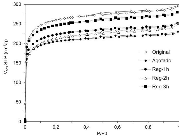
Figura 3: gráfica de las isothermas de adsorción-desorción de nitrógeno a -196^{\circ}\text{C} de un experimento de regeneración electroquímica de carbón activado agotado. Los símbolos representan: (rombo hueco con línea continua) es el carbón activado original, (rombo relleno con línea discontinua) es el carbón activado agotado, (círculo relleno con línea discontinua) es el carbón activado tomado en la primera hora de tratamiento, (triángulo hueco con línea discontinua) es el carbón activado tomado en la segunda hora de tratamiento y (cuadrado relleno con línea de puntos) es el carbón activado tomado en la tercera hora de tratamiento.
