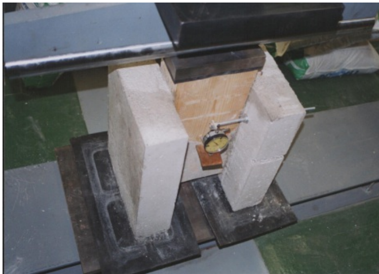
Figura 6. Probeta de conexión durante y después de su rotura.
